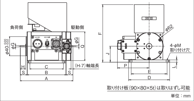
回転検出器取り付け図
