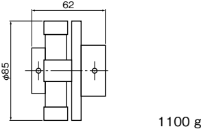
図2.センタフレックスカップリング CF-A-002-O2
