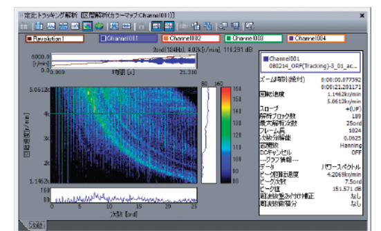
カラーマップ(定比トラッキング)
