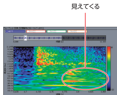
機械工作異音のウェーブレット変換結果 (時間—周波数カラースペクトル)
