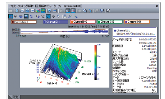
ウォーターフォール表示(定比トラッキング)
