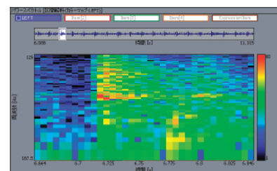
機械工作異音のFFT解析結果 (時間—周波数カラースペクトル)
