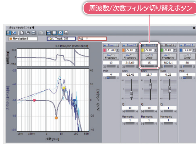
パラメトリック・イコライザ
