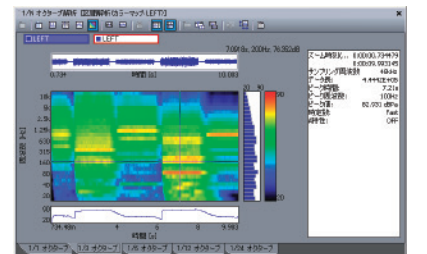
1/3オクターブ カラーマップ
