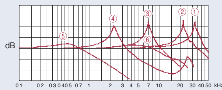
接触共振周波数特性(例)
