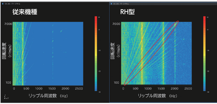
検出器違いによる比較結果例 (モータ直結構成でのトラッキング解析)
