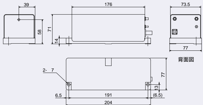
センサヘッド LV-0911
