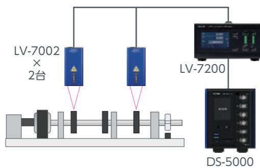
製品構成例
