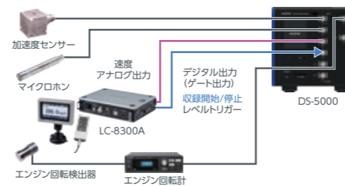
製品構成例
