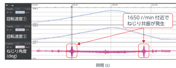
時間波形
