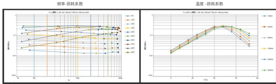
减震材料单体的损耗系数计算结果
