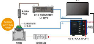
LV-1800 激光多普勒振动测量仪
