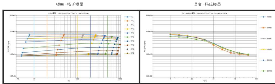
减震材料单体的杨氏模量计算结果
