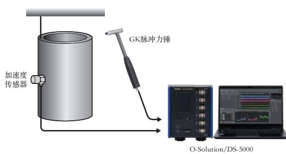
〔测量频率响应函数（例）〕
