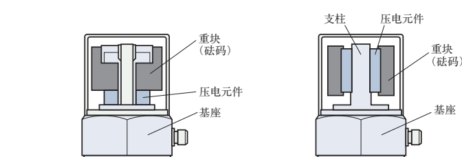
图1 压电型加速度传感器的结构
