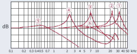
接触共振频率特性(例)
