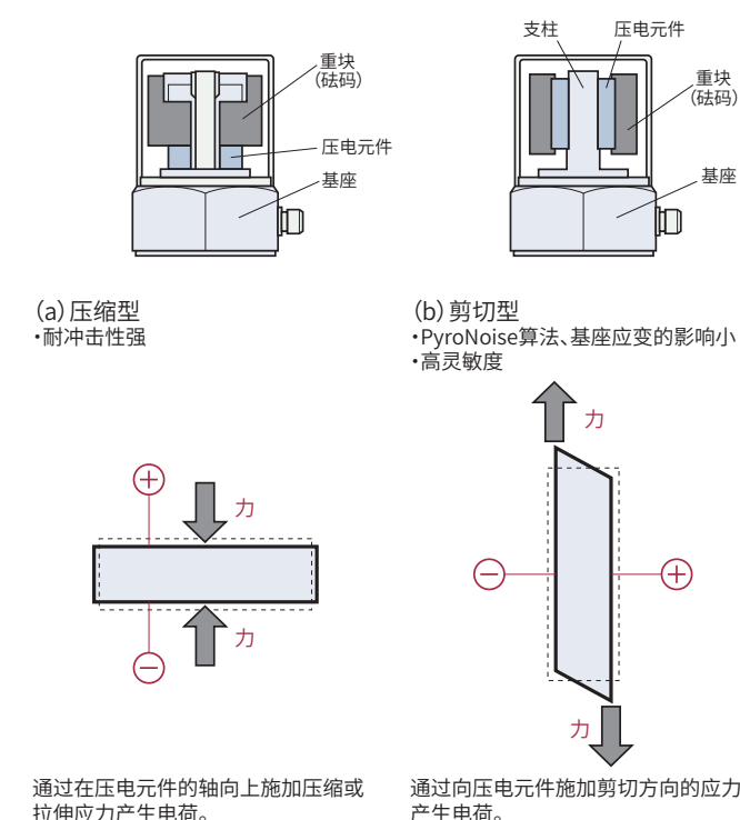
图1 压电型加速度传感器的结构
