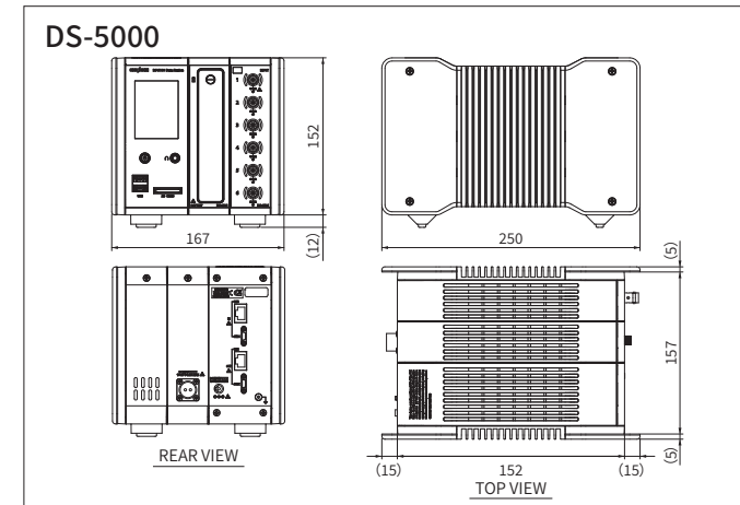
外形尺寸图 (单位:mm) ②
