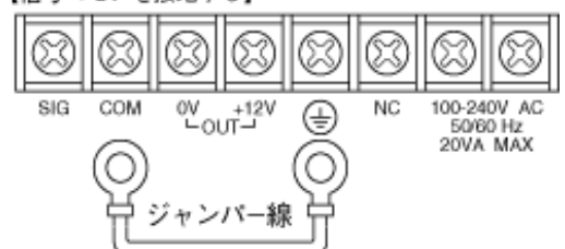
【信号コモンを接地する】
