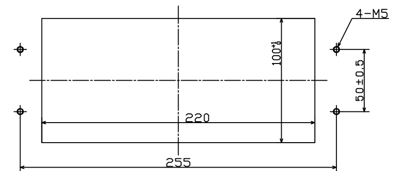
パネルカット寸法図
