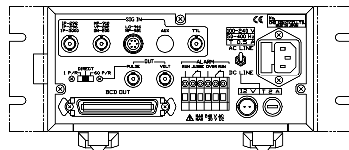
背面図
