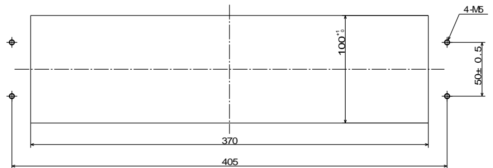
パネルカット寸法図
